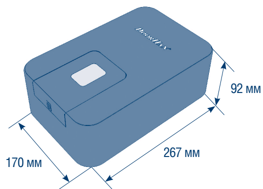
Рис. 1.2. Габаритные размеры
